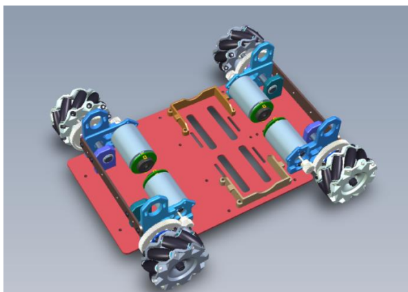
▲ 图 7.1.4 H 型车模
