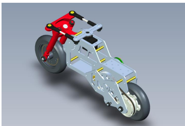
▲ 图 7.1.5 K 型车模
