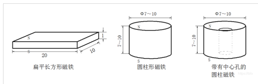
▲ 图 7.3.1 用作计时磁标的永磁铁
