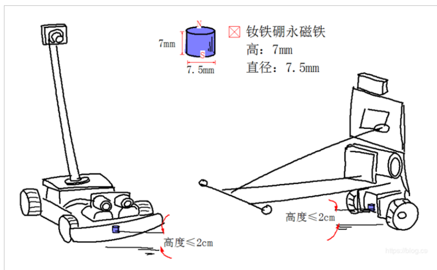
▲ 图 3.3.2 车模上安装的永磁计时磁标
