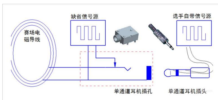
▲ 图 3.1.4 外接信号源接口示意图
