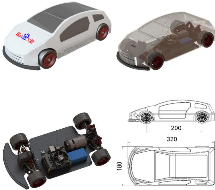
▲ 图 A7.1.10 I 车模示意图
