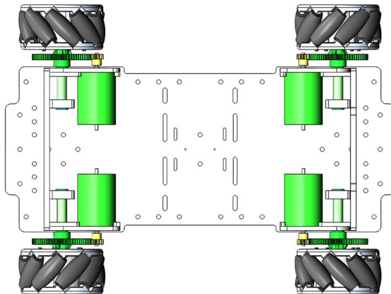
▲ 图 7.1.10 M 车模底盘
