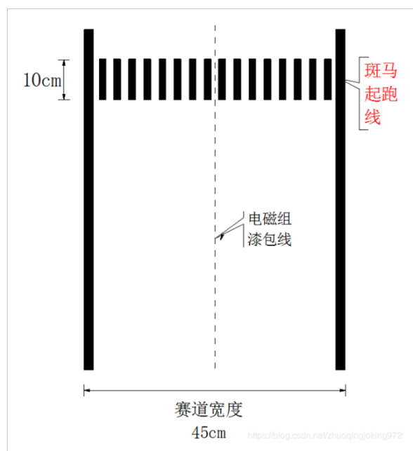
▲ 图 3.1.6 斑马起跑线
