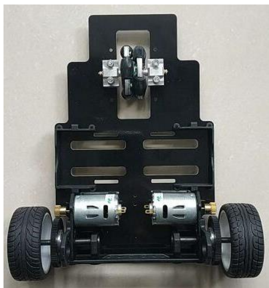
▲ 图 7.1.3 G 型车模
