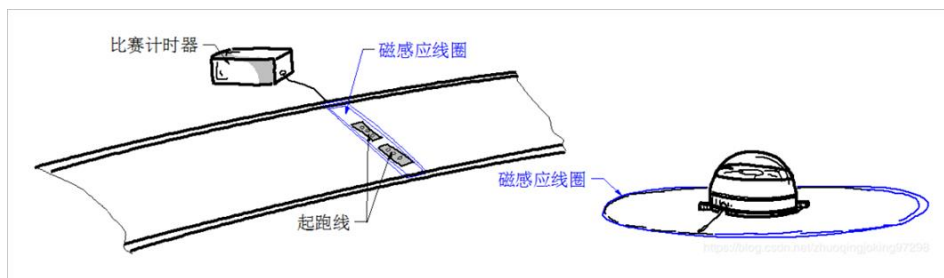
▲ 图 3.3.1 基于电磁感应的计时系统
