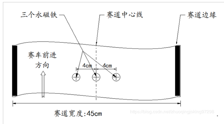
▲ 图 3.1.7 永久磁铁标志
