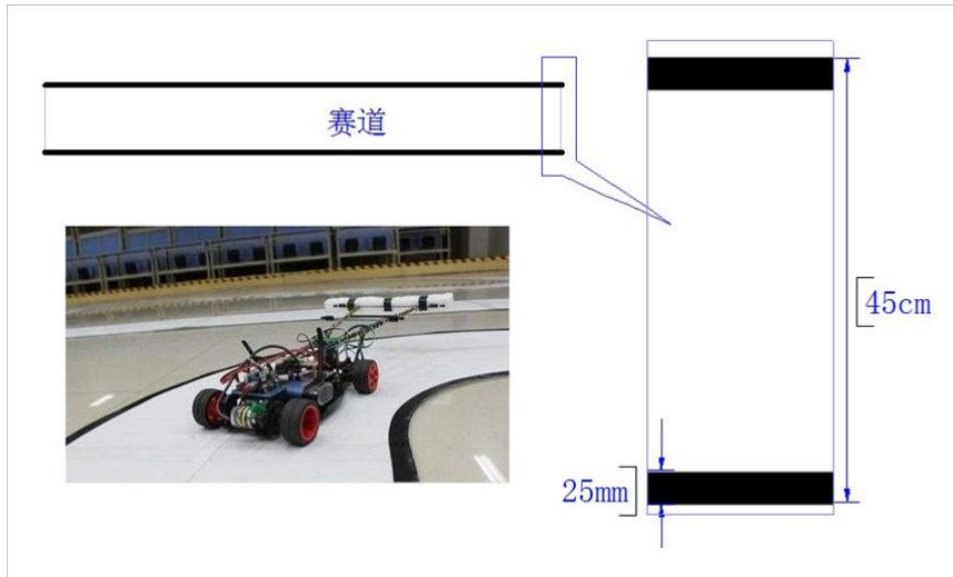
▲ 图 3.1.2 赛道边界线引导
