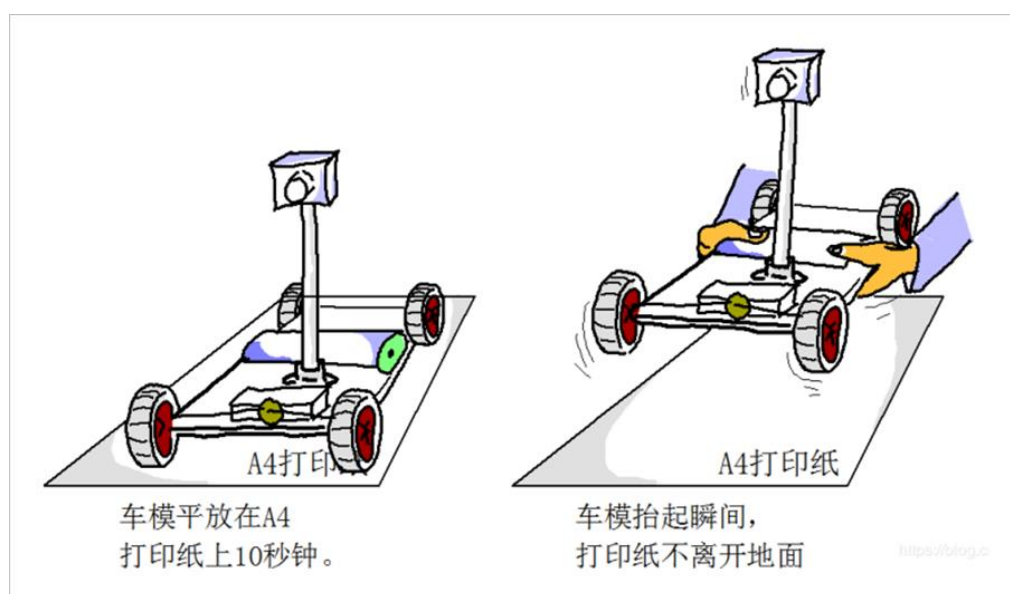
▲ 图 7.2.1 车模轮胎粘性检查
