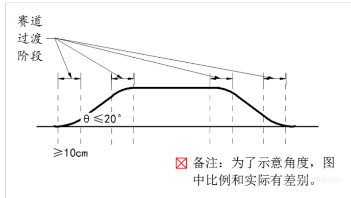
▲ 图 3.1.12 坡道示意图
